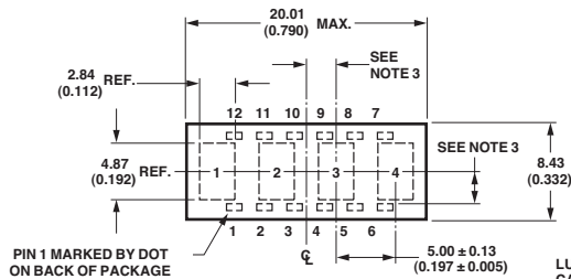
HDLx-3416
