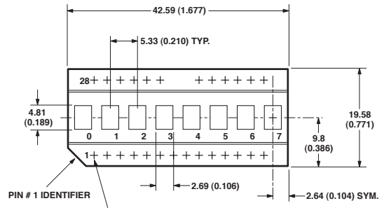
HDSP-2107,-211x
