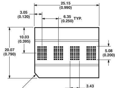
HDLx-2416
