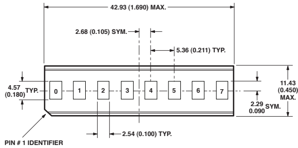
HDSP-253x
