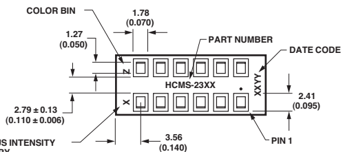
HDLx-3416
