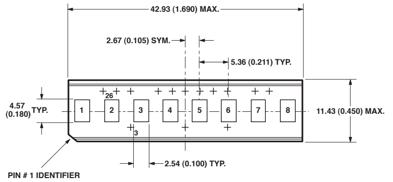
HCMS-297x/HCMS-397x
