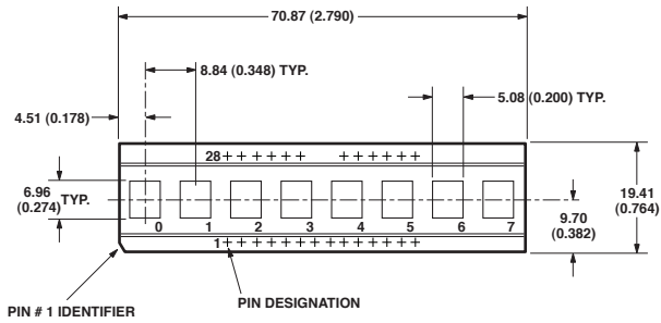
HDSP-250x
