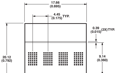
HDLx-2416
